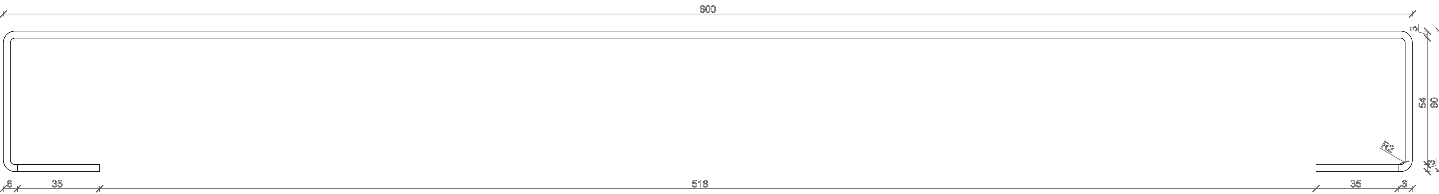
widok od spodu
