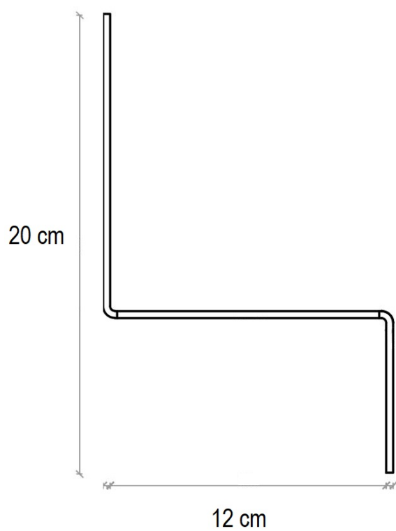
widok z prawej
